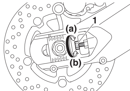
1. Einstellschraube des Antriebskettendurchhangs
