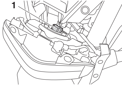
1. Scheinwerfer-Steckverbinder
