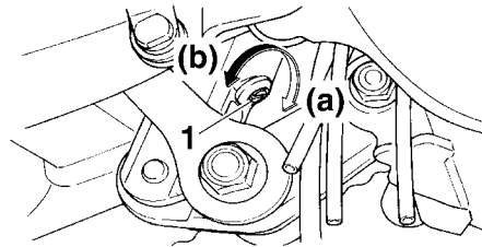
1. Zugstufendämpfungs-Einstellschraube
