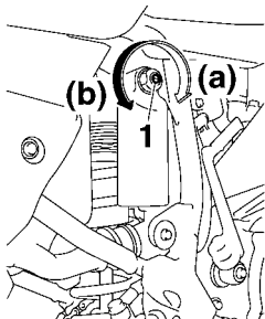
1. Druckstufendämpfungs-Einstellschraube
