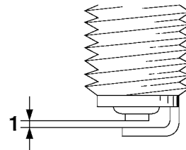
1. Zündkerzen-Elektrodenabstand
