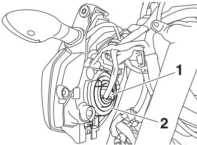
1. Fiche rapide de phare 2. Protection de l'ampoule de phare
