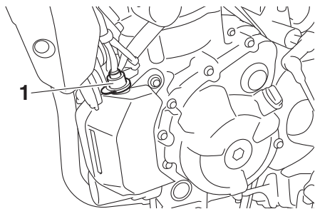
1. Kühflüssigkeits-Ausgleichsbehälterdeckel
