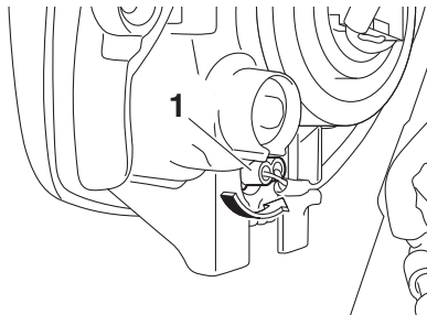
1. Cavo portalampana della luce di posizione
