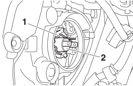
1. Portabombillas del faro 2. Bombilla del faro
