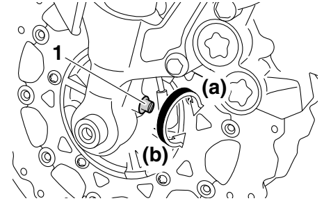
1. Vite di regolazione dello smorzamento in compressione
