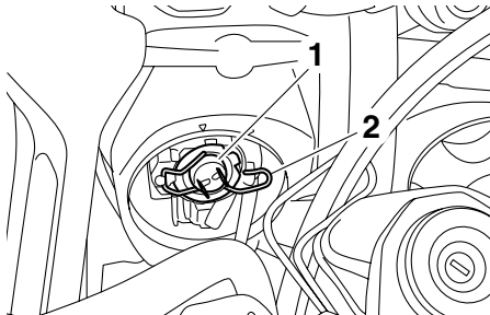
1. Lâmpada do farol dianteiro 2. Suporte da lâmpada do farol dianteiro
