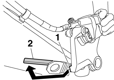
1. Retenue 2. Fente
