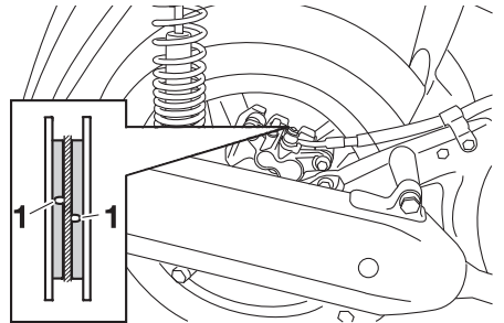
1. Verschleißanzeigerille des Bremsbelags
