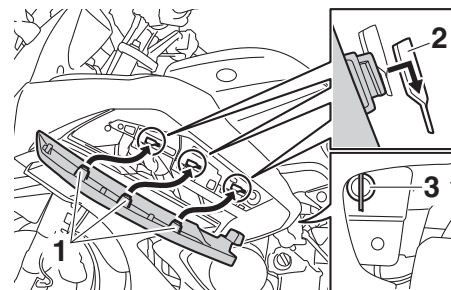
1. Vorsprung 2. Obere Aufnahme 3. Schnellverschluss
