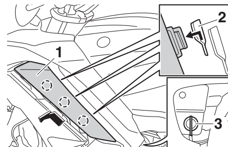
1. Abdeckung der Verkleidungs-Ventilationsöffnung 2. Untere Aufnahme 3. Schnellverschluss
