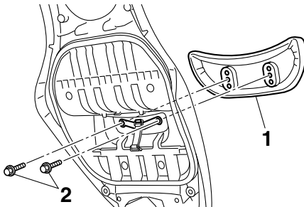
1. Fahrer-Rückenlehne 2. Schraube
