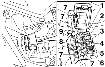
Per XP500
