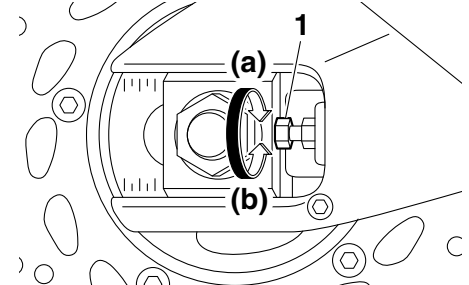
1. Cavilha ajustadora da folga da corrente de transmissão
