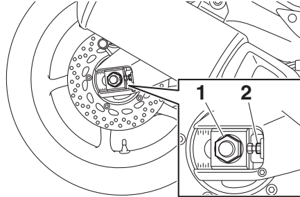
1. Porca do eixo 2. Contraporca
