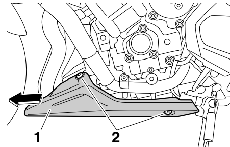
1. Carenagem A 2. Cavilha
