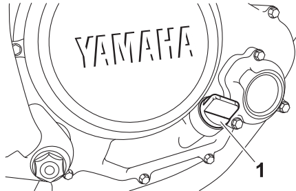
1. Motoröl-Einfüllschraubverschluss
