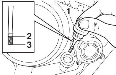
1. Motoröl-Einfüllschraubverschluss
