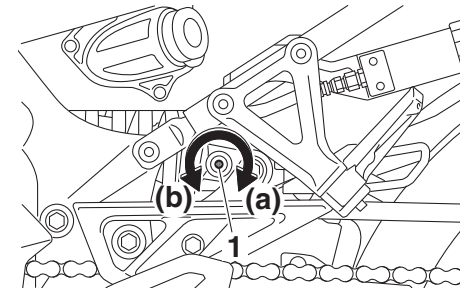
1. Einstellschraube (Zugstufen-Dämpfungskraft)
