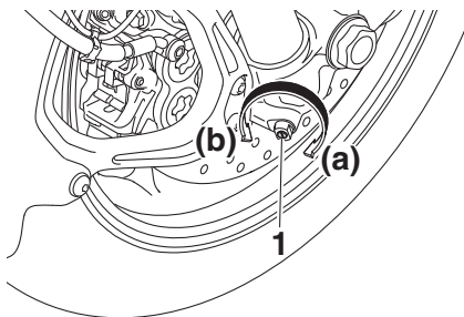
1. Druckstufendämpfungs-Einstellschraube
