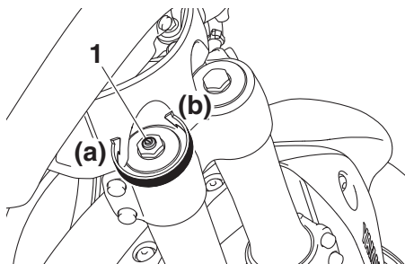
1. Einstellschraube (Zugstufen-Dämpfungs-kraft)
