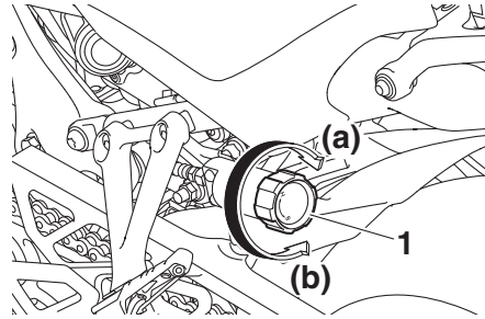
1. Mando de ajuste de la precarga del muelle
