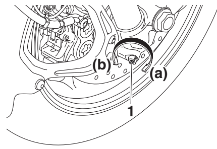
1. Tornillo de ajuste del hidráulico de compresión
