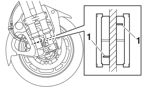
1. Slijtage-indicatorgroef remblok
