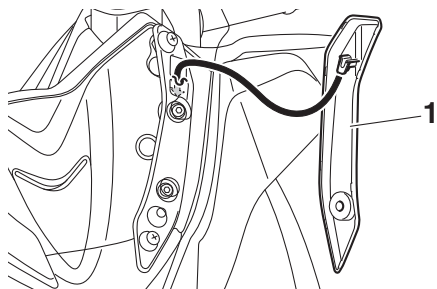
1. Coperchio di accesso ai bulloni
