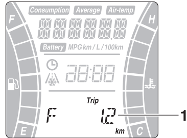
1. Contachilometri riserva
