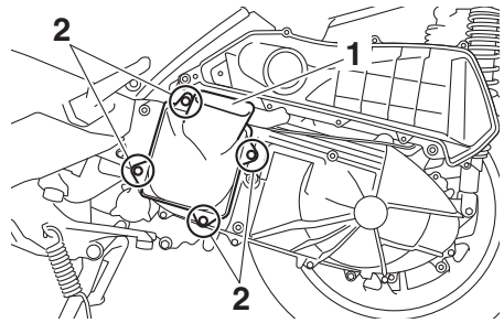
1. Coperchio cassa filtro carter cinghia trapezoidale 2. Bullone
