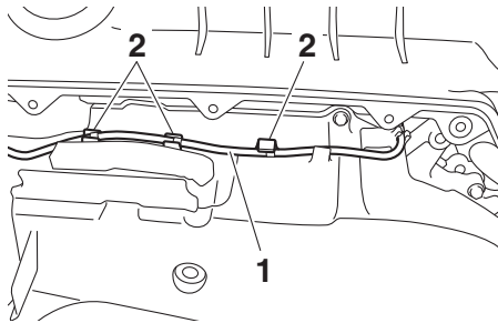
1. Cavo sensore ruota posteriore 2. Supporto per cavo
