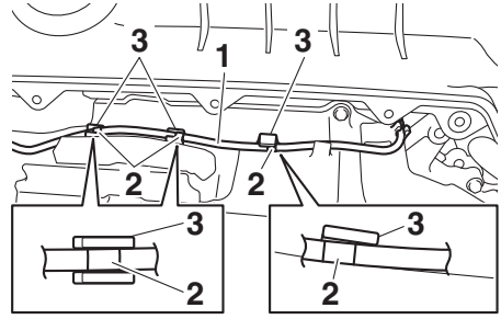
1. Bedrading achterwielsensor
