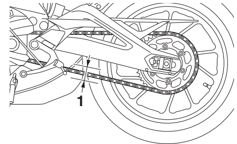
1. Antriebsketten-Durchhang
