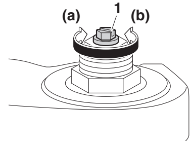
1. Einstellschraube (Zugstufen-Dämpfungskraft)
