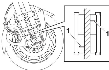
1. Slijtage-indicatorgroef remblok
