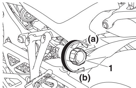
1. Stelknop veervoorspanning
