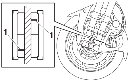
1. Slijtage-indicatorgroef remblok
