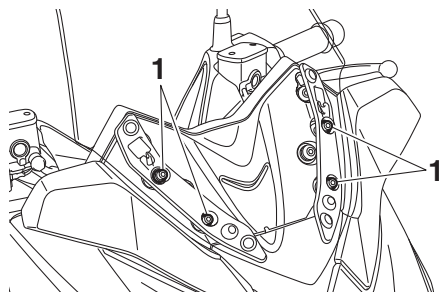
1. Cavilha
