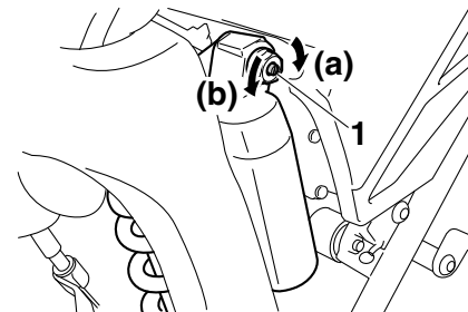
1. Druckstufendämpfungs-Einstellschraube
