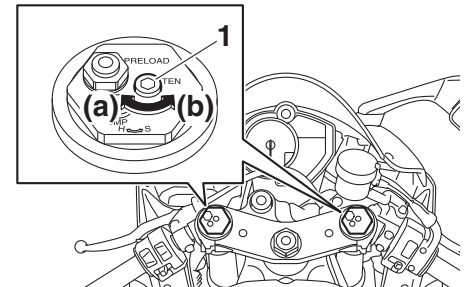
1. Perno de ajuste de la amortiguación en extensión
