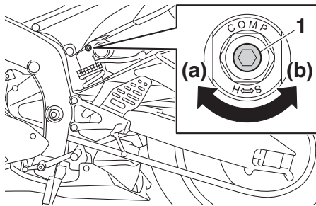
1. Justerbult för långsam kompressionsdämning
