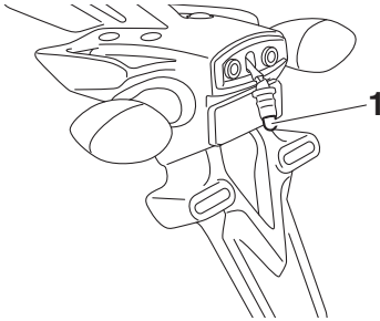
1. Lâmpada da luz da chapa de matrícula
