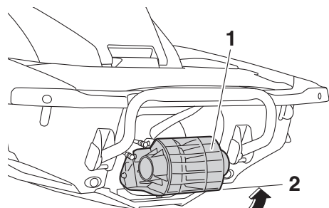
1 Inverseur 2 Point mort
