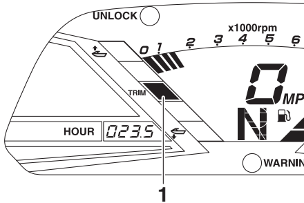
1 Ενδεικτικό ζυγοστάθμισης
