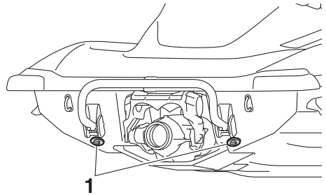
1 Τάπα αποστράγγισης πρύμνης
