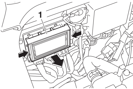
1 Sicherungskastenabdeckung
