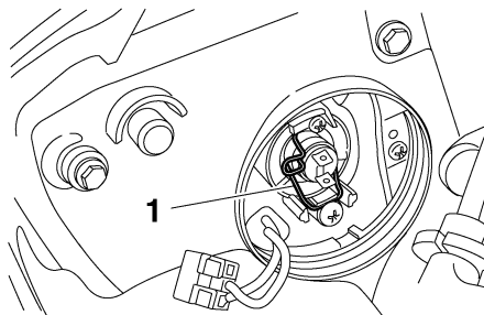
1. Gloeilamphouder
