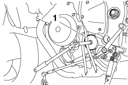
1. Oliefiltersleutel
