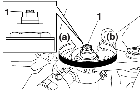
1. Stelschroef voor uitgeerdemping
