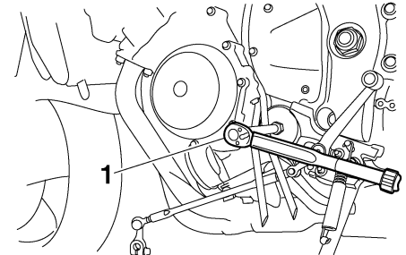
1. Momentsleutel
