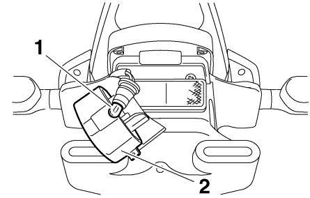
1. Lâmpada da luz da chapa de matrícula 2. Unidade da luz da chapa de matrícula
