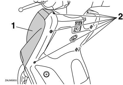
1. Verkleidungsteil A
