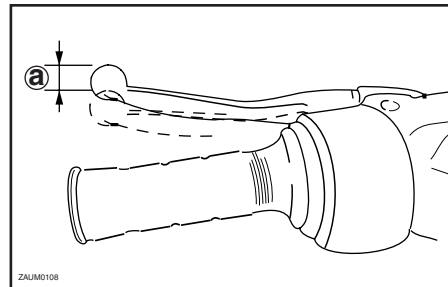
a. Hinterradbremshelmspiel
