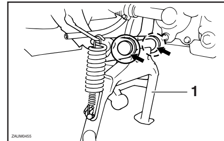
1. Hauptständer
