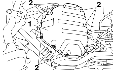
1. Luftfiltergehäuseabdeckung 2. Schraube
