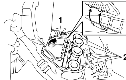
1. Luftfiltereinsatz 2. Einlasskrümmer
