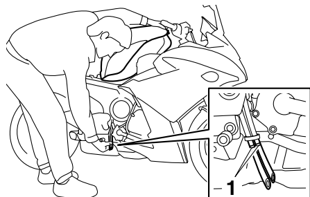
1. Ausgangsstellung (Farbmarkierung)
