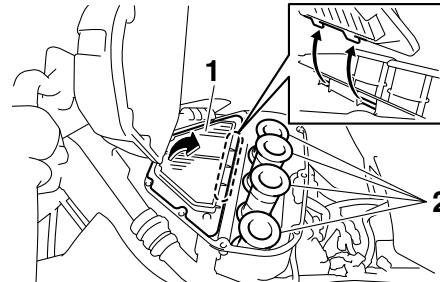
1. Luftfiltereinsatz 2. Einlasskrümmer
