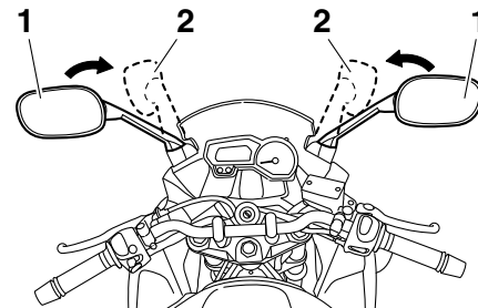
1. Fahrposition 2. Parkposition
