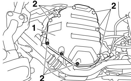
1. Tampa da caixa do filtro de ar 2. Parafuso
