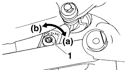
1. Zugstufendämpfungs-Einstellschraube
