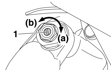
1. Druckstufendämpfungs-Einstellschraube (für langsame Dämpfung)
