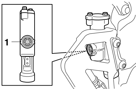
1. Minimalstand-Markierung
