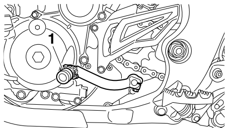
1. Pedale cambio
