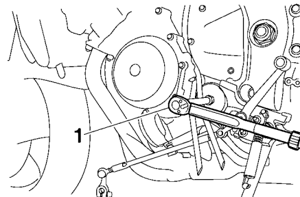
1. Clé dynamométrique
