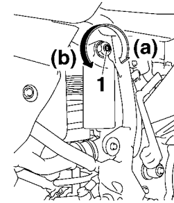
1. Druckstufendämpfungs-Einstellschraube
