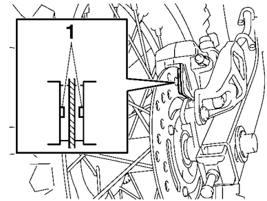
1. Verschleißanzeiger des Bremsbelags
