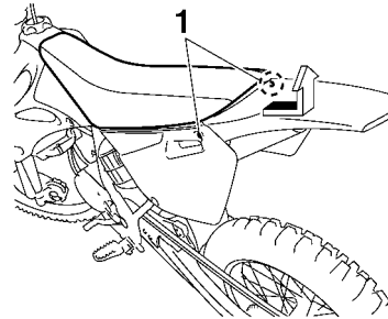
1. Schraube
