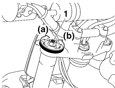
1. Zugstufendämpfungs-Einstellschraube
