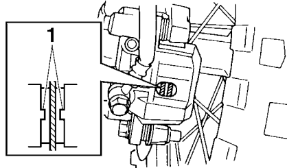
1. Verschleißanzeiger des Bremsbelags
