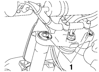
1. Entlüftungsschraube
