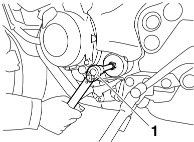
1. Momentsleutel
