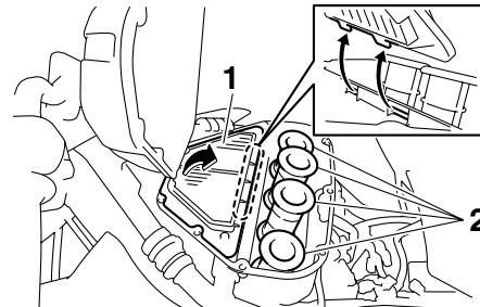
1. Luchtfilterelement 2. Luchtinlaatspruitstuk
