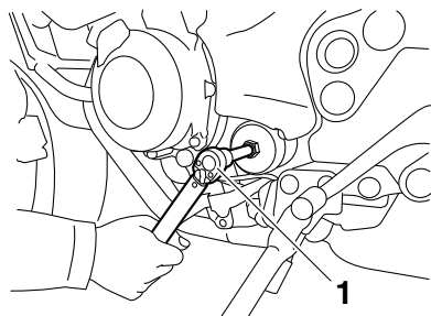
1. Chiave dinamometrica
