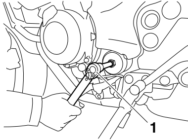
1. Momentnyckel
