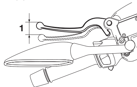
1. Garde du levier de frein
