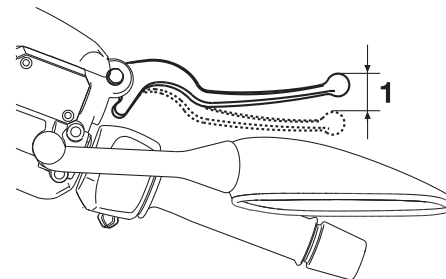
1. Folga da alavanca do travão
