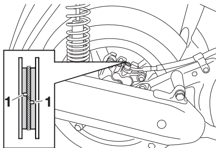
1. Ranhura indicadora de desgaste da pastilha do travão
