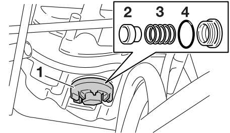
1. Vis de vidange d'huile moteur B
